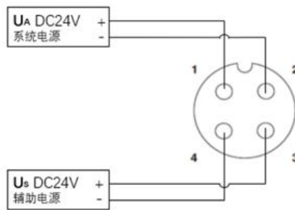
电源端口
